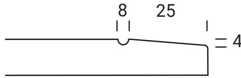
Edge Profile
